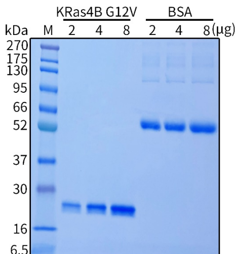
图2. 碧云天Recombinant Human KRas4B (G12V, His-Tag) (P2413)的SDS-PAGE电泳检测图。本蛋白经BeyoGel™ Plus PAGE 预制胶(Tris-Gly, 4-15%, 10孔) (P0465)电泳, Marker为BeyoColor™彩色预染蛋白分子量标准(6.5-270kD) (P0071/P0072), 并经BeyoBlue™考马斯亮蓝超快染色液(P0017F)染色。实际检测结果可能会因样品和检测条件等的不同而存在差异, 图中数据仅供参考。
